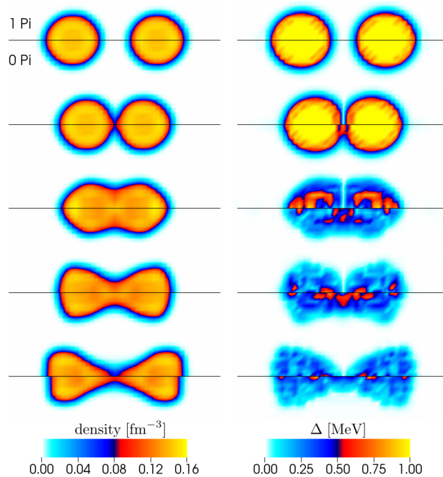
Figure 1: Dynamika jądrowa w ramach TDSLDA: Rysunek przedstawia czołowe zderzenie ^{240}\text{Pu}+^{240}\text{Pu} o niskiej energii. Lewa kolumna przedstawia całkowite rozkłady gęstości nukleonów w jądrach, a prawa - rozkłady gęstości par Coopera, odpowiedzialnych za nadciekłość. Część górna każdego rysunku odpowiada zderzeniu z kreacją wzbudzenia solitonowego powstającego pomiędzy jądrami (prawa kolumna).
